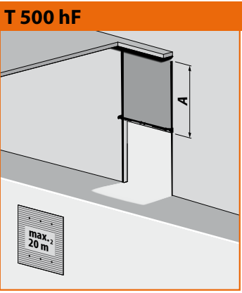
Schienensystem mit Vertikalführung, mit unten liegender Federwelle + Stahl-Trageprofil A = lichte Höhe + 400 mm Breite max. 4500 mm
