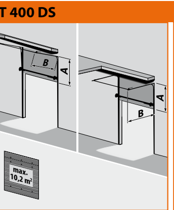
Schienensystem mit Höherführung, mit unten liegender Federwelle A = Hebung + 200 mm B = lichte Höhe - Hebung + 600 mm Breite max. 3200 mm Höhe max. 3200 mm Hi-lift min. 1700 mm
