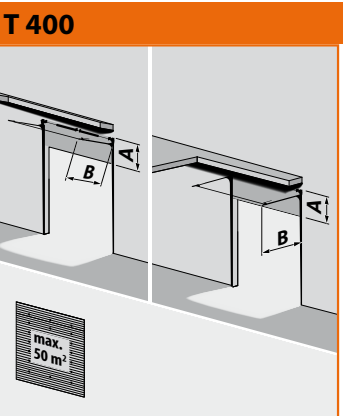
Schienensystem mit Höherführung A = Hebung + 400 mm B = lichte Höhe - Hebung + 600 mm
