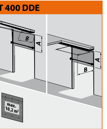
Federloses Schienensystem mit Vertikalführung A = Hebung + 200 mm B = lichte Höhe - Hebung + 600 mm Breite max. 3200 mm Höhe max. 3200 mm Hi-lift min. 1700 mm
