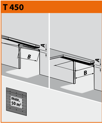
Schienensystem mit Normalführung (Standard) A = 430-510 mm B = lichte Höhe + 650 mm
