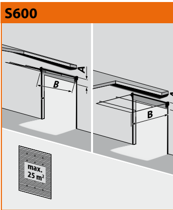
Helix S600 Horizontale Schienensystem A = 600 mm B = lichte Höhe + 265 mm Breite max. 5000 mm
