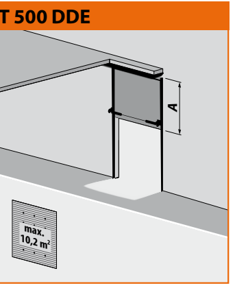
Federloses Schienensystem mit Vertikalführung A = lichte Höhe + 400 mm Breite max. 3200 mm Höhe max. 3200 mm
