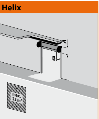
Helix Spiral A = 1100 mm B = 1200 mm Breite max. 5000 mm Höhe: min. 2500 mm max. 5000 mm
