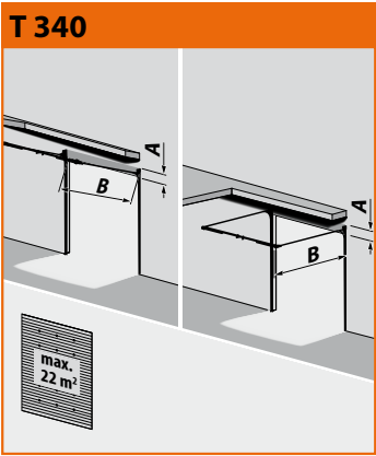
Schienensystem mit Normalführung, Federaggregat hinten + Stahl-Trageprofil A = 340 mm B = lichte Höhe + 750 mm Breite max. 6500 mm
