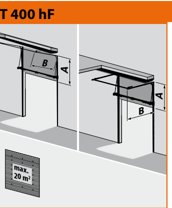
Schienensystem mit Höherführung, mit unten liegender Federwelle + Stahl-Trageprofil A = Hebung + 200 mm B = lichte Höhe - Hebung + 600 mm Breite max. 4500 mm Hi-lift min. 1450 mm
