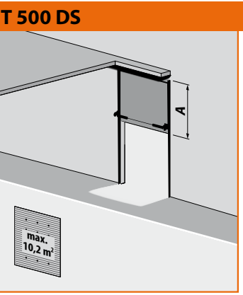
Schienensystem mit Vertikalführung, mit unten liegender Federwelle A = lichte Höhe + 400 mm Breite max. 3200 mm Höhe max. 3200 mm
