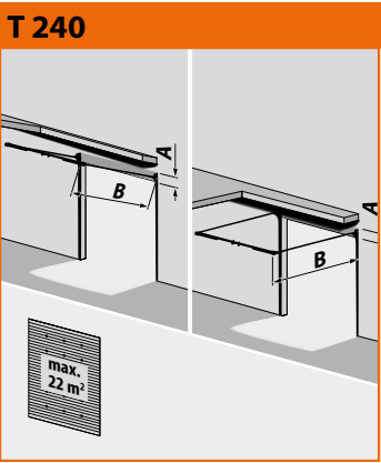
Niedrigsturz-Schienensystem, innenliegende Drahtseile + Stahl-Trageprofil A = 240 mm B = lichte Höhe + 1.000 mm Breite max. 6500 mm
